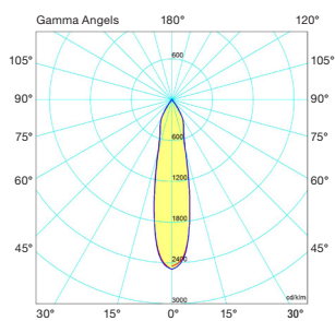
LYSKURVER 20W 60°
