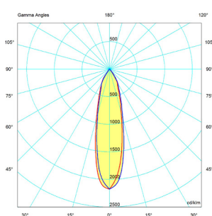
LYSKURVER 40W 60°
