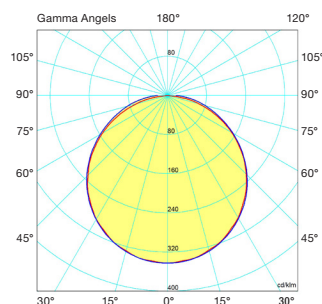
LYSKURVER 200W
