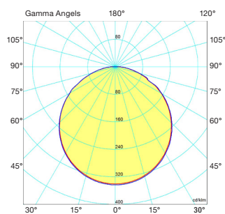
LYSKURVER 120W (120cm)
