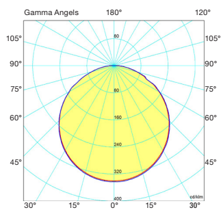
LYSKURVER 120W (90cm)
