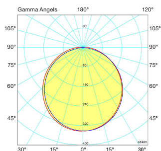
LYSKURVER 160W
